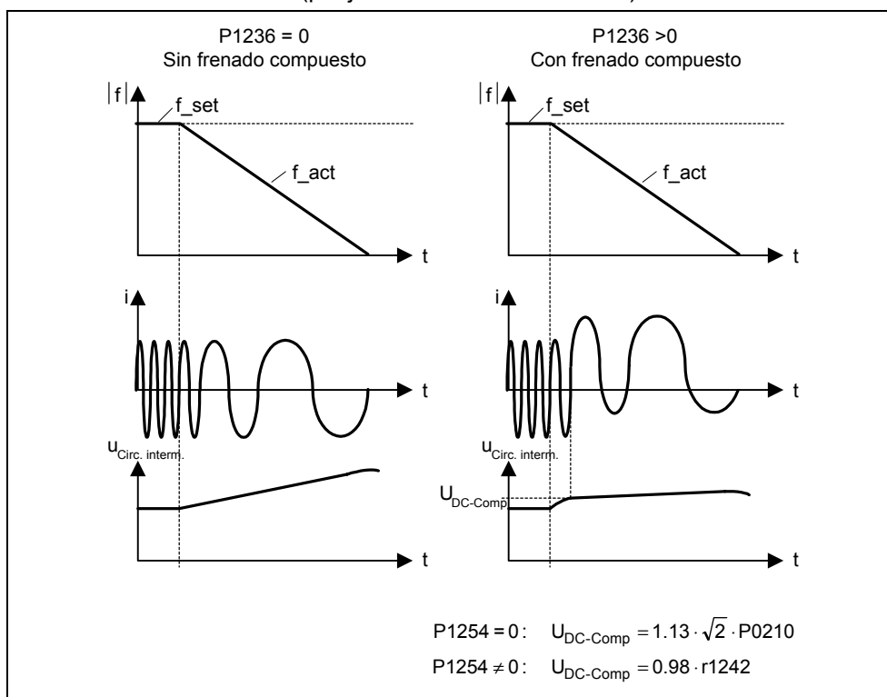
Figura 3-53 Freno combinado
