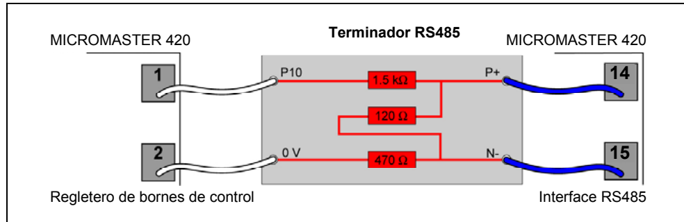
Figura 3-30 Terminador RS485
