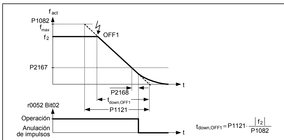
Figura 3-44 OFF1
