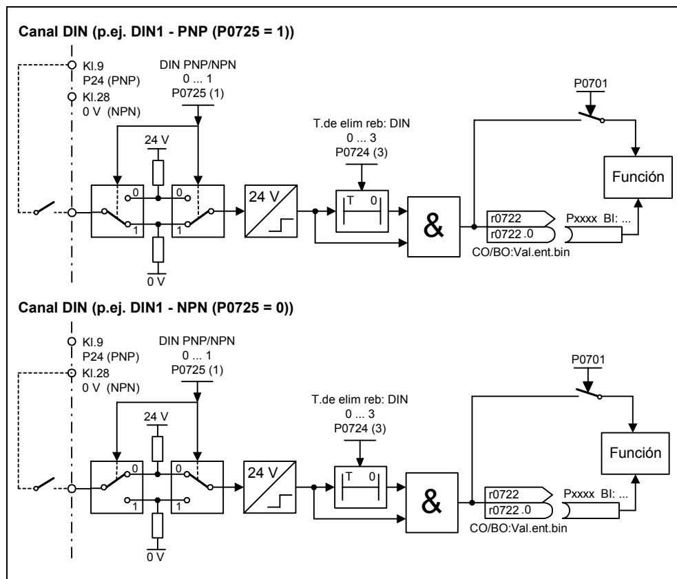
Figura 3-22 Entradas digitales
