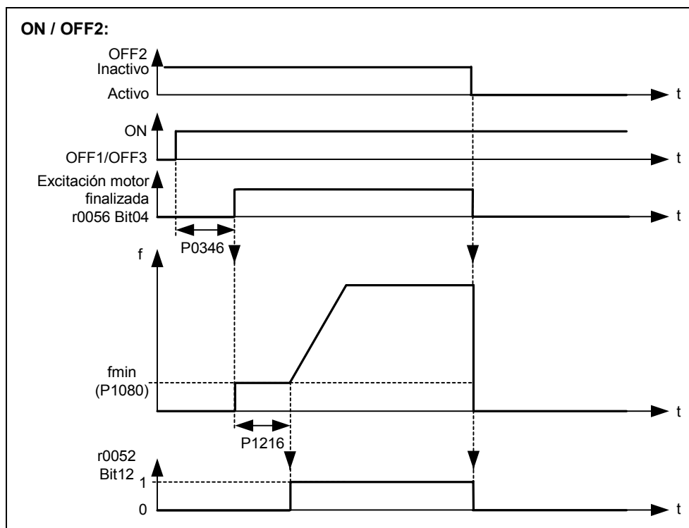
Figura 3-49 Freno de mantenimiento del motor por OFF2
