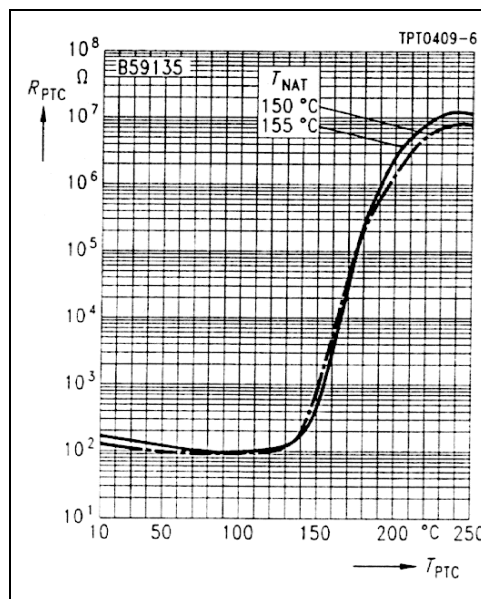
Figura 3-57 Curva característica del PTC para motores 1LG y 1LA
