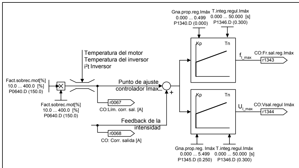
Figura 3-64 Regulador Imáx.
