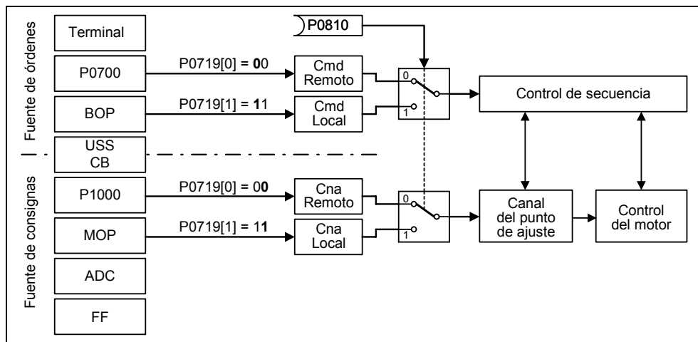
Figura 3-47 Conmutación vía parámetros BICO P0810
