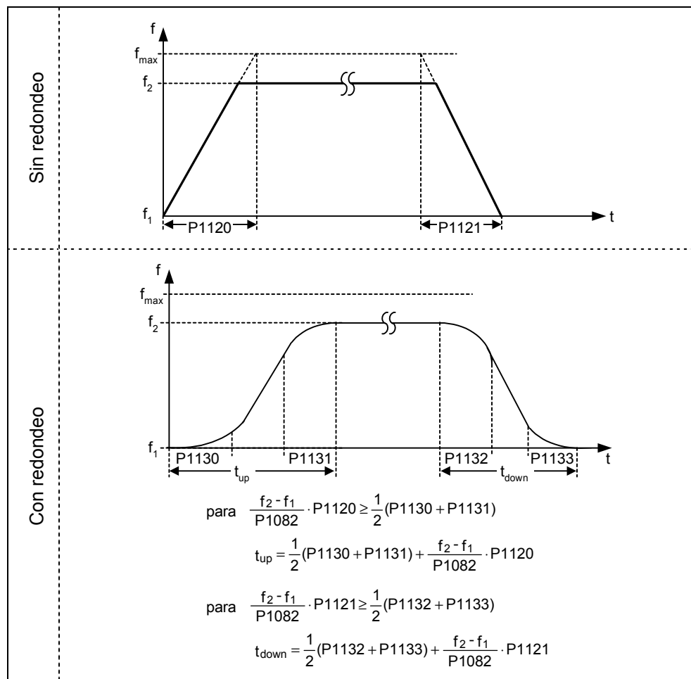
Figura 3-42 Generador de rampas
