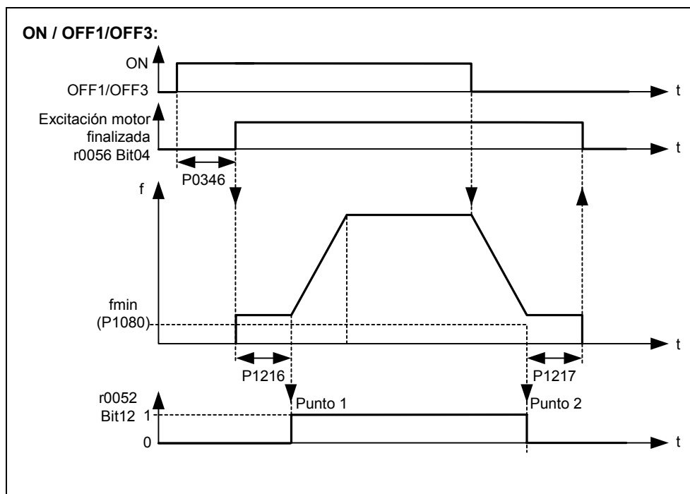
Figura 3-48 Freno de mantenimiento del motor después de ON / OFF1
