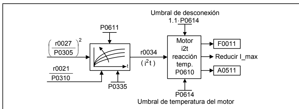
Figura 3-56 Reacciones del convertidor
