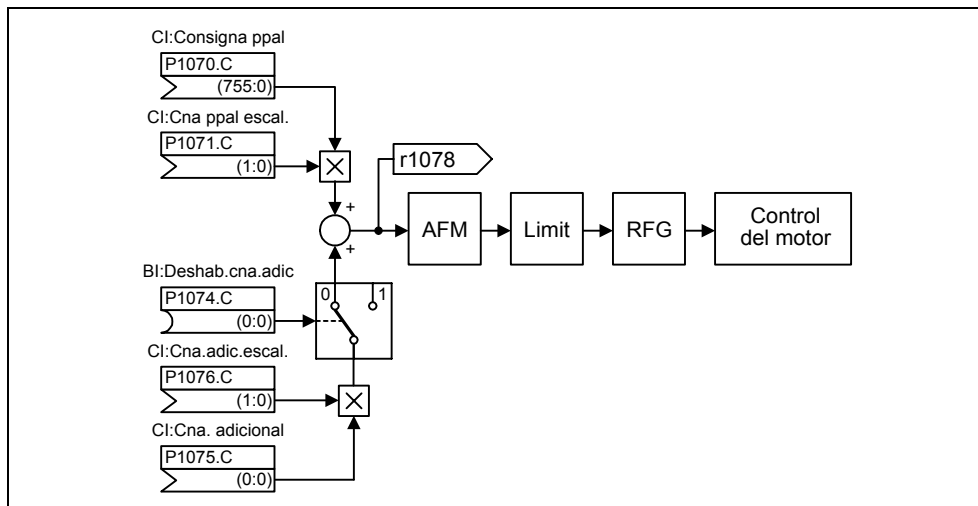
Figura 3-40 Suma de consignas
