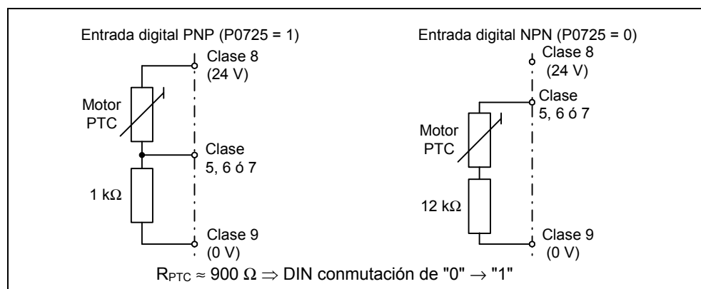
Figura 3-58 Conexión del sensor de temperatura al MICROMASTER 420
