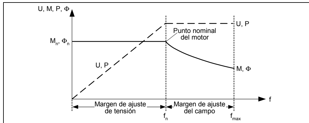
Figura 3-61 Zona operacional y desarrollo de la característica de un motor asíncrono alimentado por convertidor
