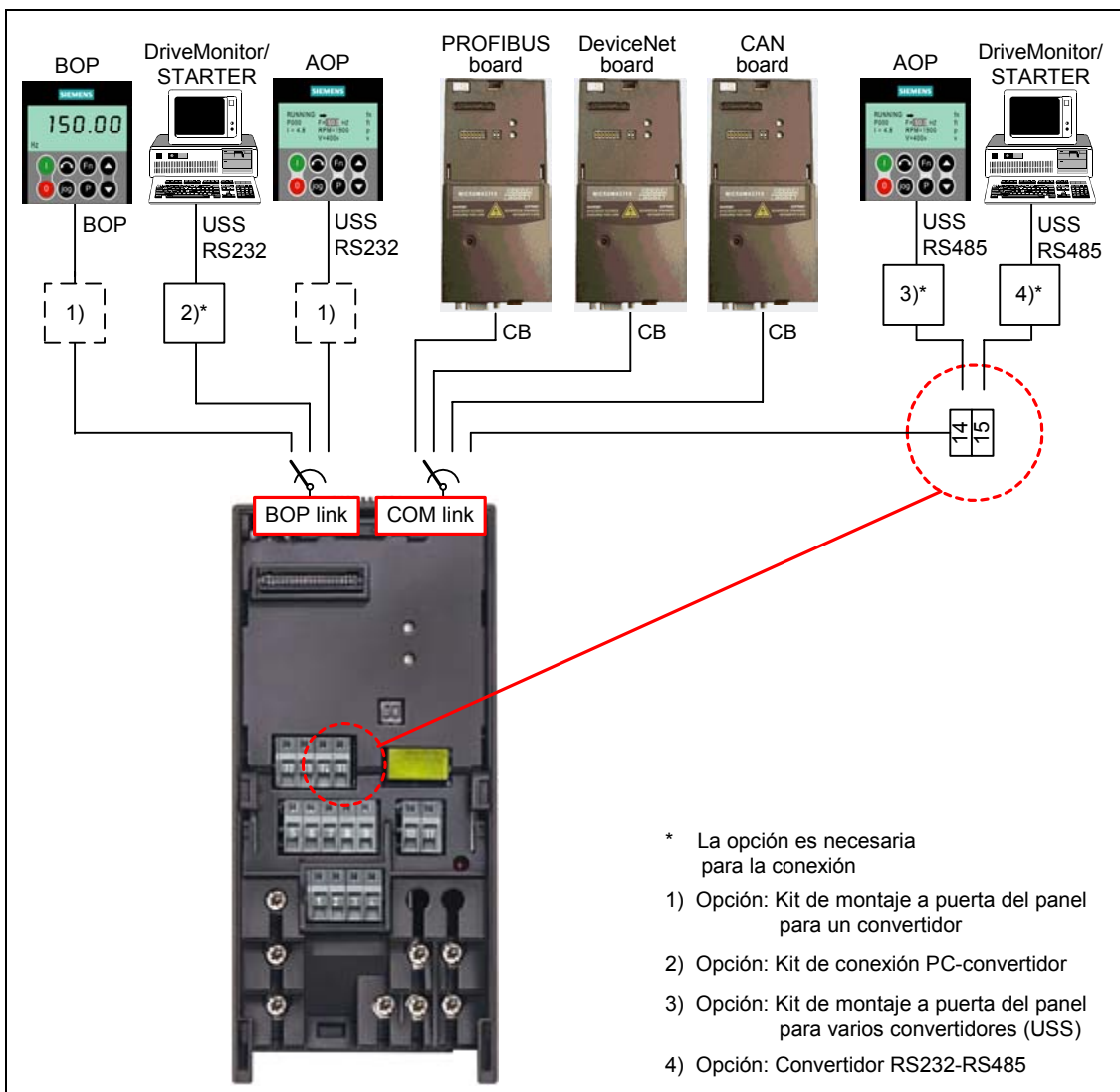
Figura 3-29 Interfaces de comunicación en serie: BOP y COM
