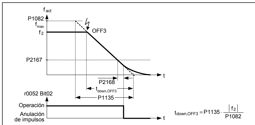
Figura 3-46 OFF3
