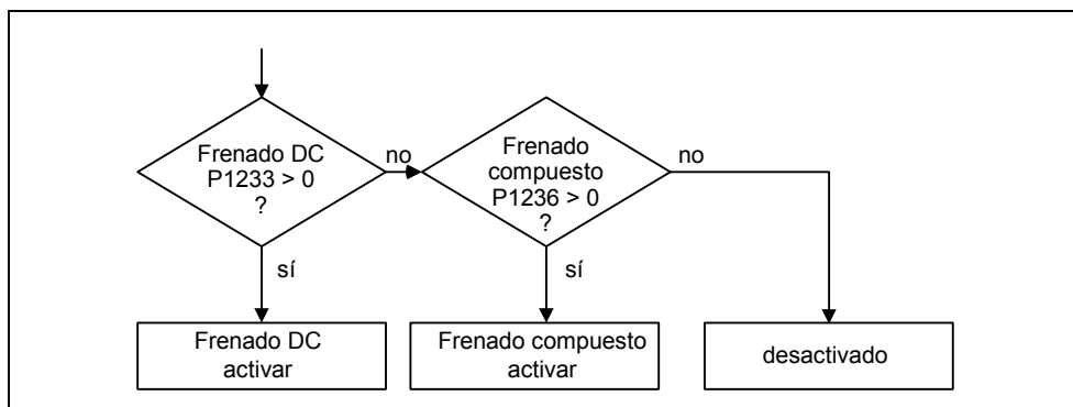
Figura 3-50 Dependencia de los frenos electrónicos.
