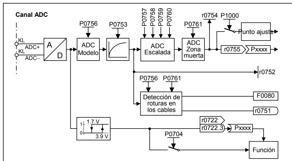
Figura 3-25 Canal ADC
