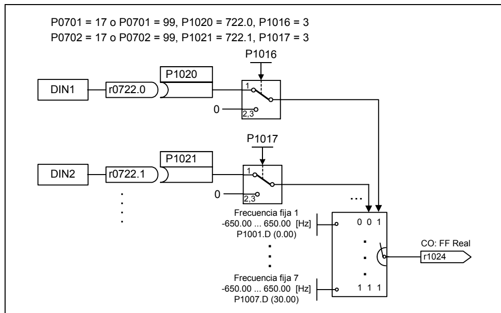
Figura 3-33 Ejemplo para selección binaria de FF1 vía DIN1 y FF2 vía DIN2
