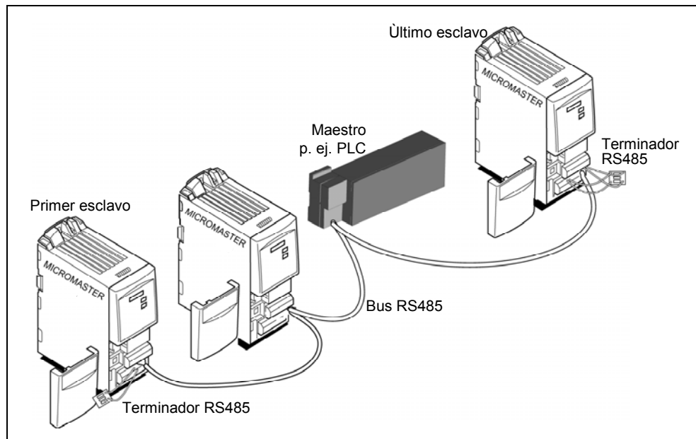
Figura 3-31 Estructura del bus USS
