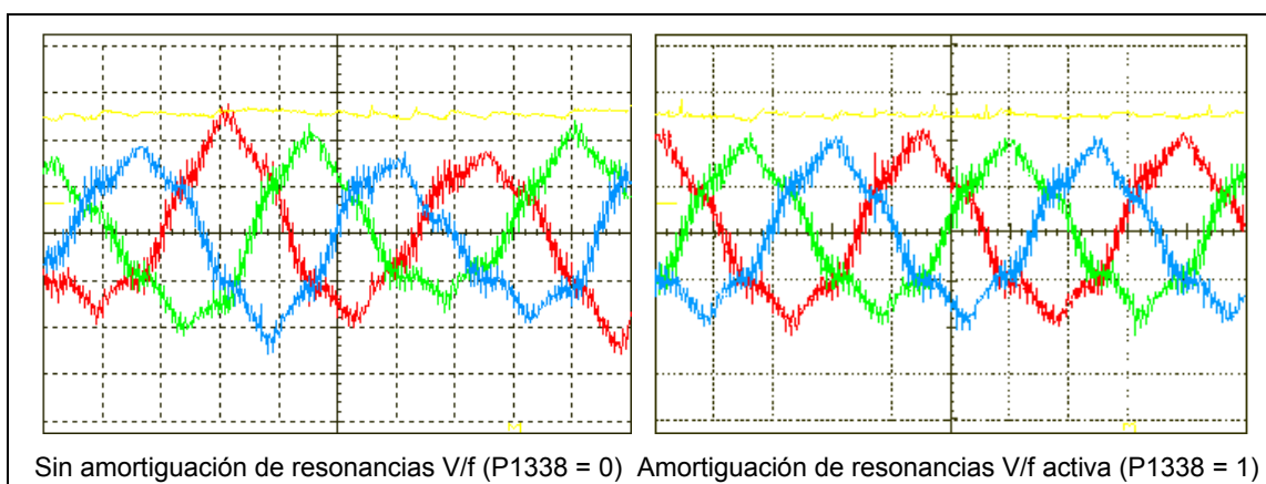
Figura 3-63 resultado de la amortiguación de resonancias V/f
