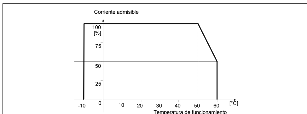
Figura 2-2 Temperatura de funcionamiento
