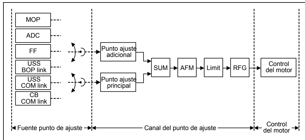
Figura 3-39 Canal de consignas
