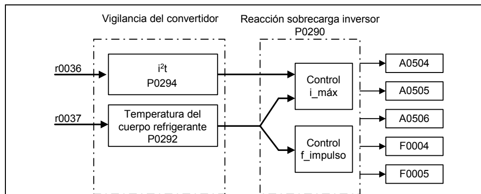
Figura 3-60 Sobrecarga del convertidor (P0290)
