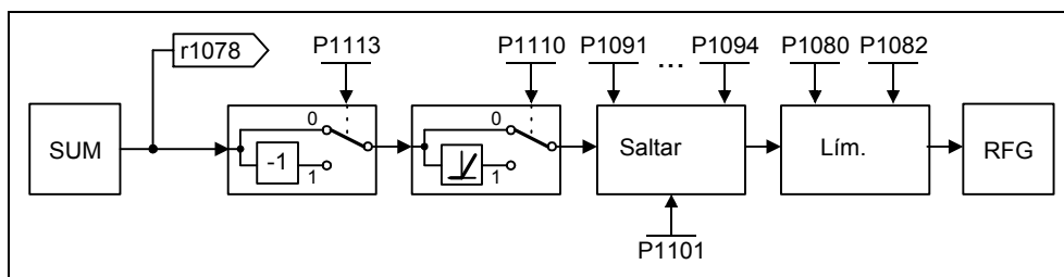
Figura 3-41 Modificación de consignas de frecuencia
