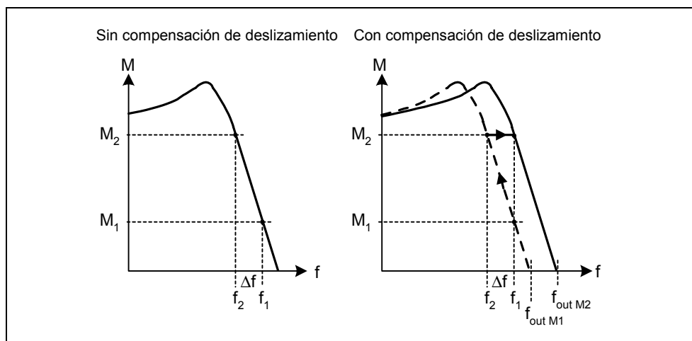
Figura 3-62 Compensación de deslizamiento
