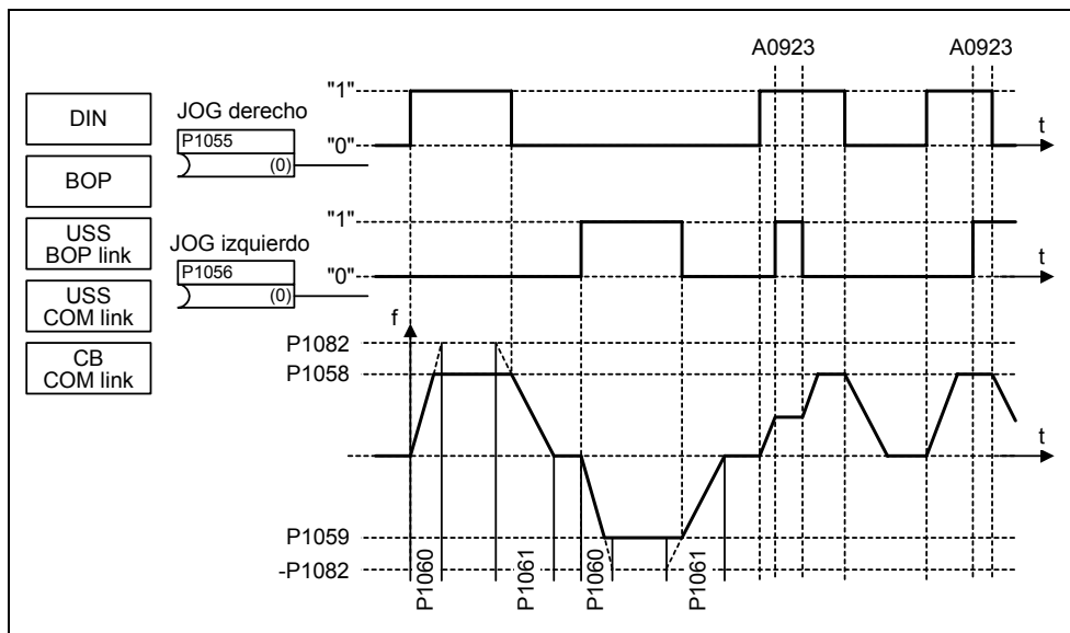
Figura 3-35 JOG izquierda o JOG derecha
