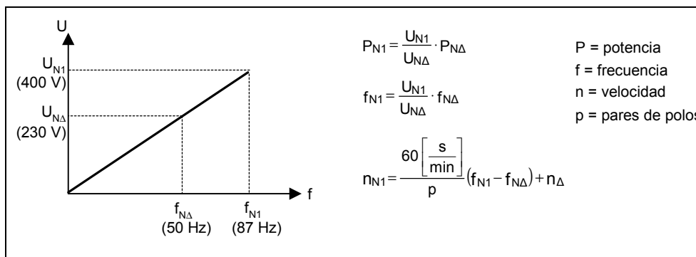
Figura 3-20 Característica V/f
