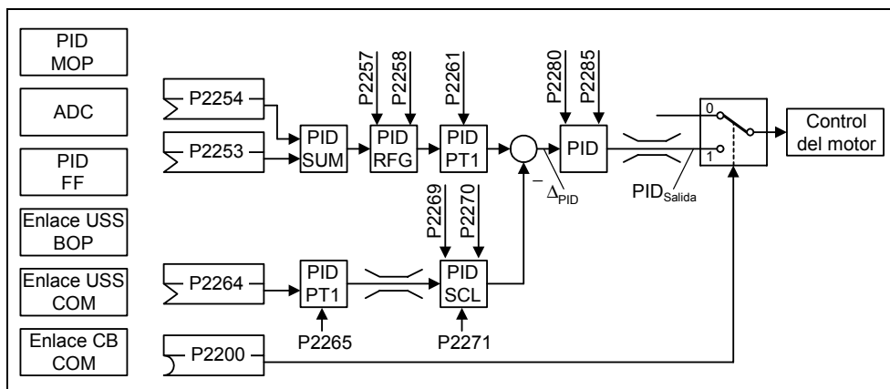
Figura 3-36 Estructura del regulador tecnológico (regulador PID)
