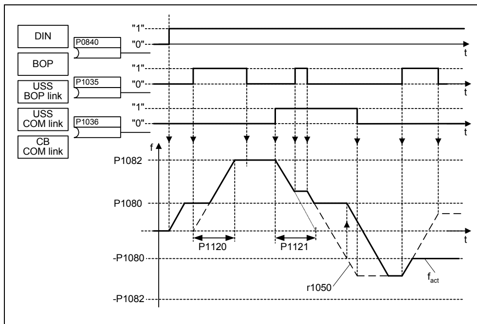
Figura 3-34 Potenciómetro motorizado
